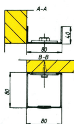
Karmtyp A2 Utanpåliggande montage. Sidostycke av fyrkantsprofil. Överstykke av u-profil.
