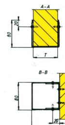
Karmtyp D Monteras på en montageprofil. Överstycket anpassas till väggjockleken (T).
