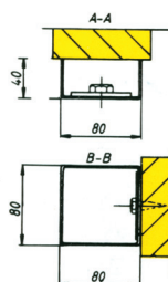
Karmtyp A Sidostycke av fyrkantsprofil. Överstykke av u-profil.
