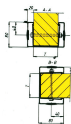
Karmtyp C Foderbildande u-profil som anpassas till väggjockleken (T). Karmen monteras med genomgående bult.
